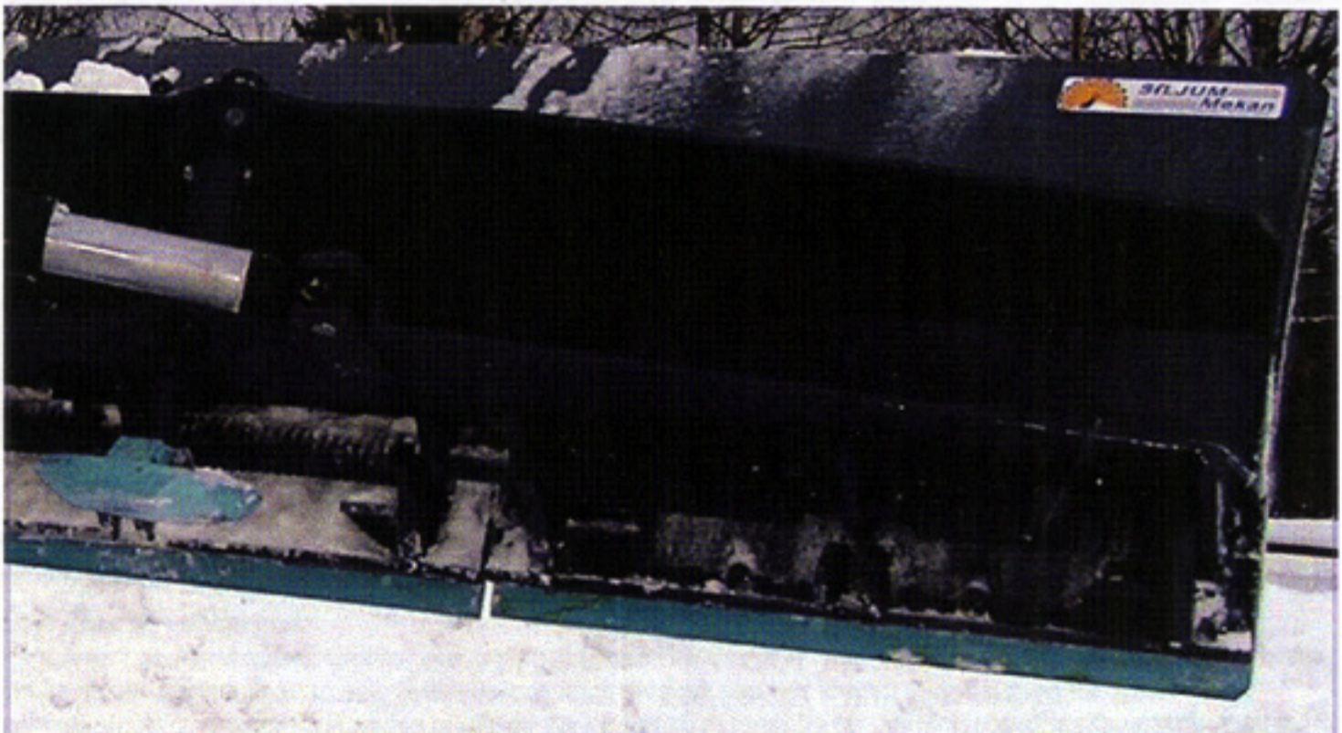
Diagonalplog sedd bakifrån. Vridfjädrar till stålhållare.
